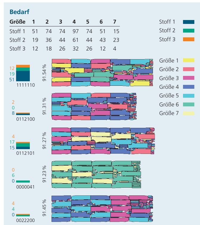
3) Lösung durch Berechnung der Materialkosten, Materialausnutzung 91,44 %, Rechenzeit: 30 Minuten
