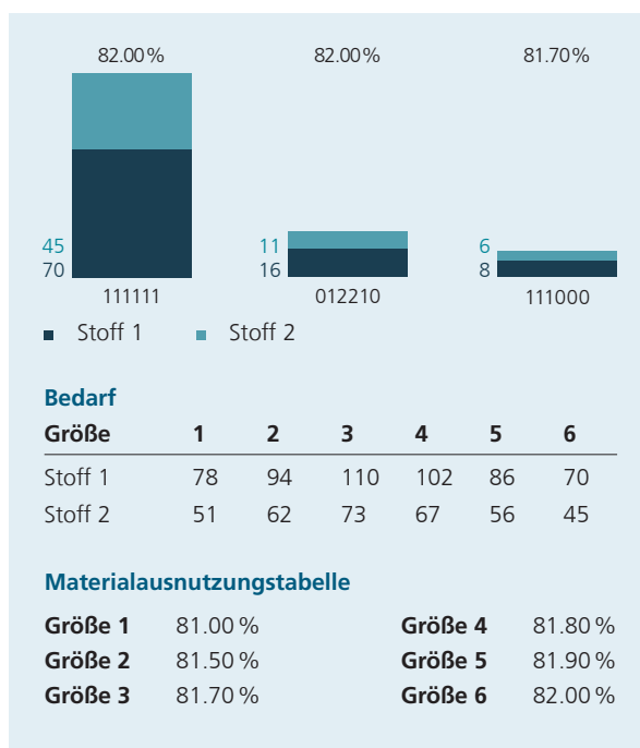
2) Lösung durch Schätzung der Materialkosten, Materialausnutzung 81,99%, Rechenzeit: < 1 Minute
